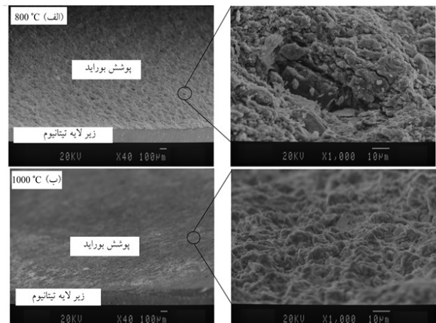
شکل ۴. ریزساختار و توپوگرافی سطح تیتانیوم بوردهی شده در دمای (الف) 800^{\circ}\text{C} و (ب) 1000^{\circ}\text{C} از زاویه مایل در دو بزرگنمایی متفاوت.
