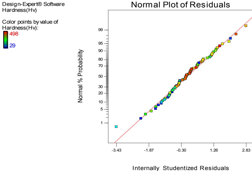
شکل ۲. منحنی احتمال نرمال باقی‌مانده برای بهینه‌سازی سختی پوشش آندایزینگ آلومینیوم.
