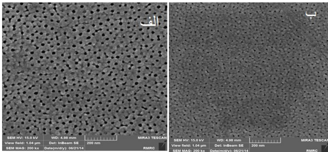
شکل ۴. تصاویر میکروسکوپ الکترونی گسیل میدانی از سطح لایه آندی الف- نمونه آندایز شده تحت جریان مستقیم با دانسیته جریان 4 \text{ A/dm}^2 ، دمای 10^\circ\text{C} و زمان 30 \text{ min} . ب- نمونه آندایز شده تحت شرایط جریان مستقیم پالس با جریان حداکثر 4 \text{ A/dm}^2 و حداقل 3 \text{ A/dm}^2 ، دمای 10^\circ\text{C} و زمان 30 \text{ min} .
