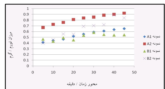
شکل ۲. نمودار میزان جذب نمونه‌های اصلی در محلول بافر pH=۴
