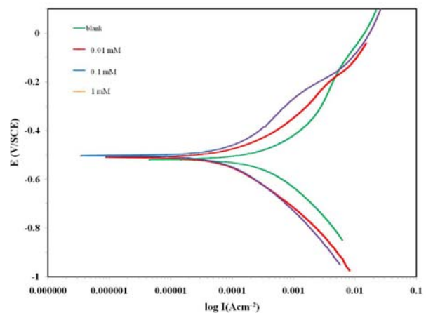
شکل ۲. منحنی‌های پلاریزاسیون پتانسیودینامیک برای فولاد ساده کربنی در محیط اسیدکلریدریک نیم مولار در حضور و عدم حضور بازدارنده با غلظت‌های ۰/۰۱، ۰/۱ و ۱ میلی مولار.
