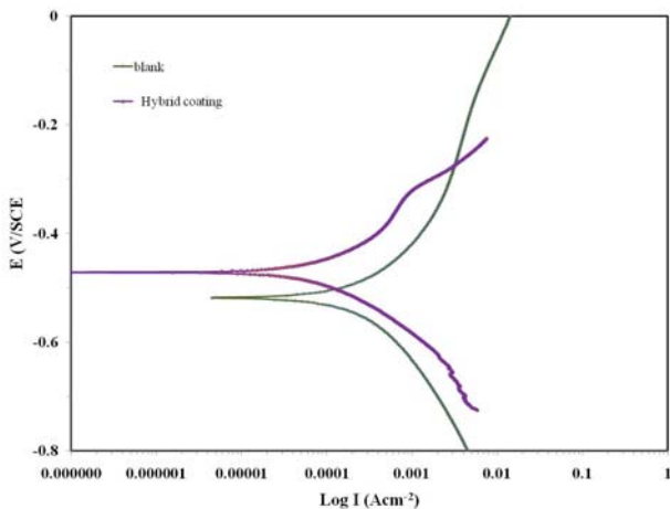
شکل ۴. منحنی‌های پلاریزاسیون پتانسیوداینامیک برای فولاد ساده کربنی با و بدون پوشش هیبریدی در محلول اسید کلریدریک نیم‌مولار.
