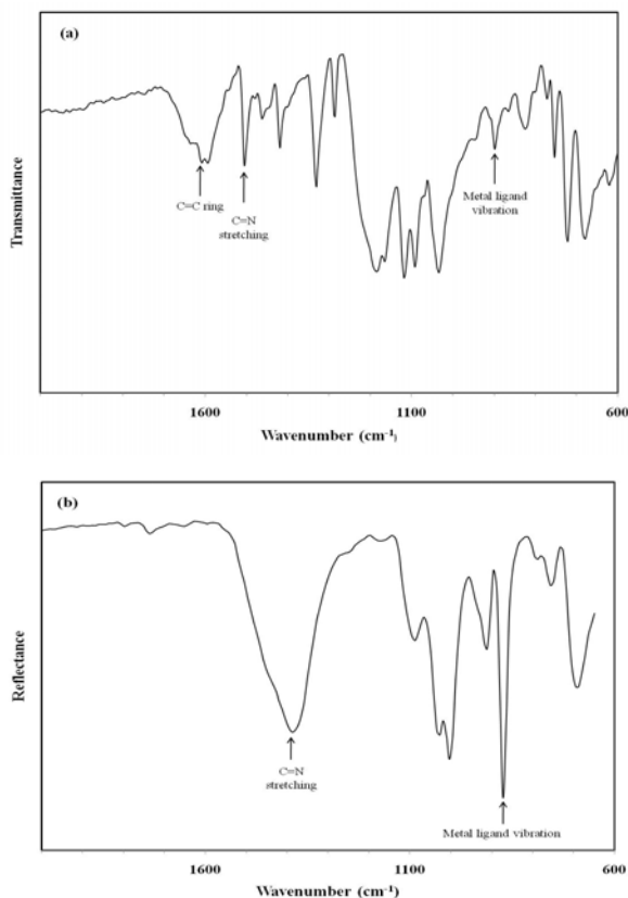
شکل ۱۰. طیف FTIR انعکاسی از فتالوسیانین مس سولفون شده جامد و لایه نازک خودمجمع فتالوسیانین مس سولفون شده.
