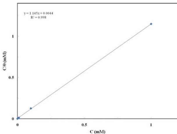
شکل ۳. ایزوترم لانگمویر برای جذب CuPh روی سطح فولاد ساده کربنی.
