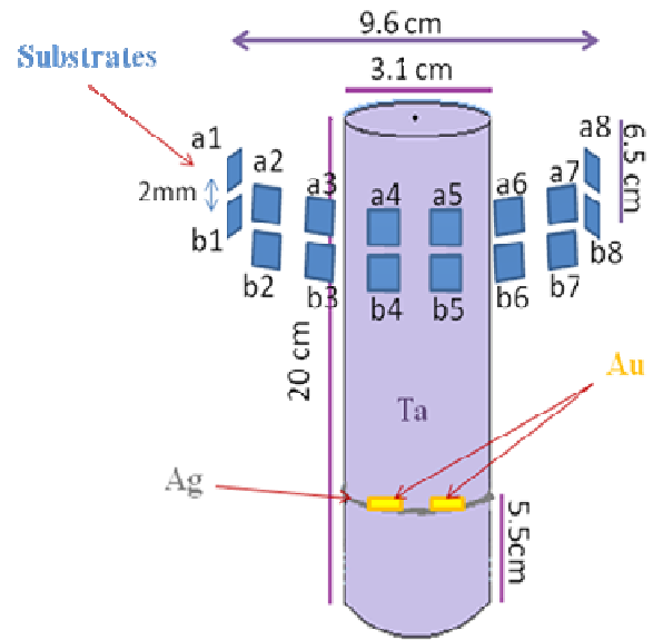
شکل ۱. شماتیک مکان قرارگیری تارگت‌ها و زیرلایه‌ها.
