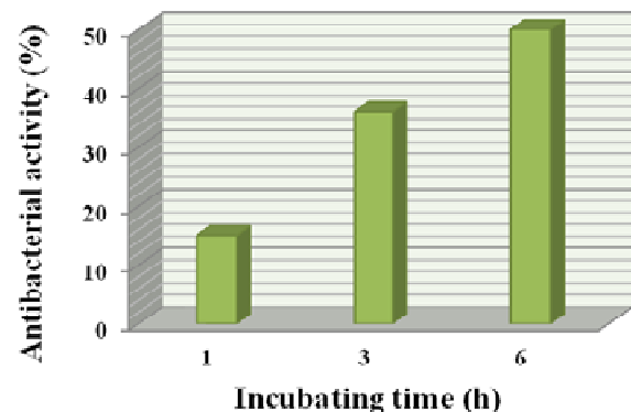
شکل ۴. نمودار نتایج فعالیت ضدباکتری لایه نیتريدانتالم - نقره/طلا برحسب مدت زمان (ساعت) تماس با سوسپانسیون باکتری.
