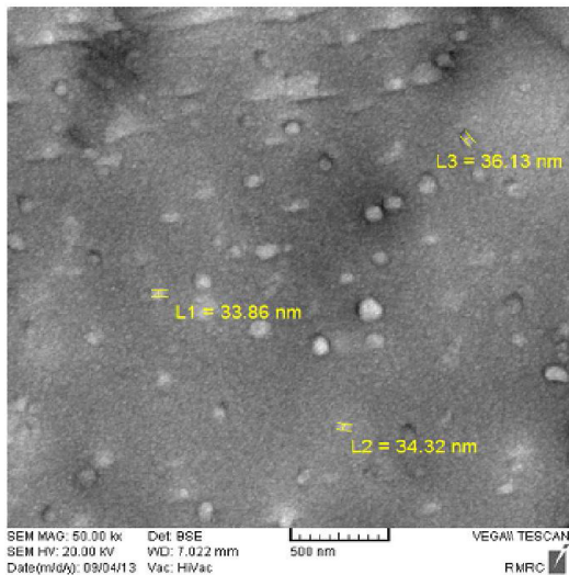
شکل ۳. تصویر میکروسکوپ الکترونی از سطح لایه نیتريد تانتالم- نقره/طلا.
