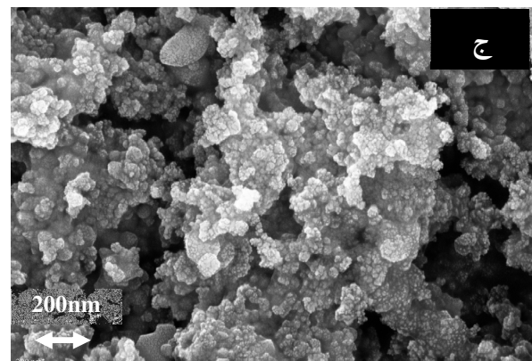
شکل ۱. تصاویر میکروسکوپی الکترونی روبشی نشر میدانی از الف: ورق تیتانیوم و نانو ذرات آلومینا با اندازه متوسط ب: ۲۰ نانومتر و ج: ۸۰ نانومتر.
