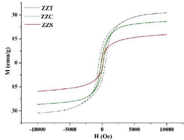
شکل ۲. منحنی‌های M-H نمونه‌های ZZT، ZZC و ZZS
