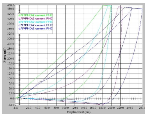
شکل ۴. نمودار نانوفروندگی پوشش کامپوزیتی
