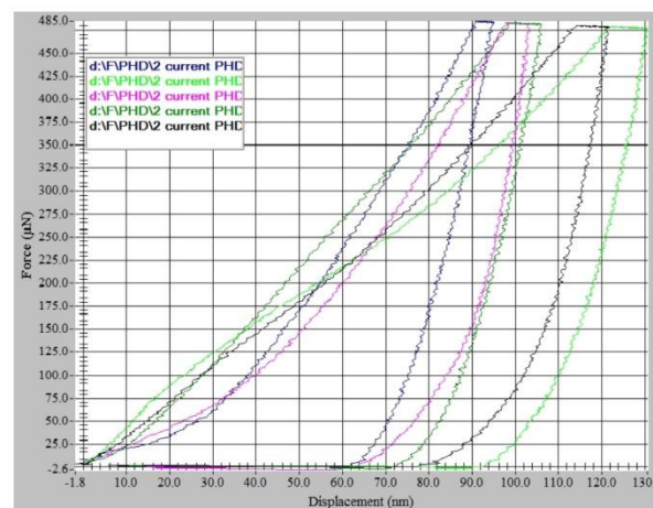
شکل ۵. نمودار نانوفروروندگی پوشش مرتبه‌ای
