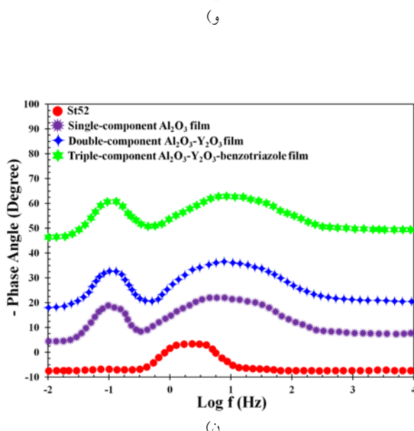
شکل ۶. نمودارهای بد و بد- فاز حاصل از آزمون EIS برای مدت زمان غوطه‌وری: الف-ب) یک ساعت، ج-د) ۴۸ ساعت، و-ن) ۹۶ ساعت [۱۴].
