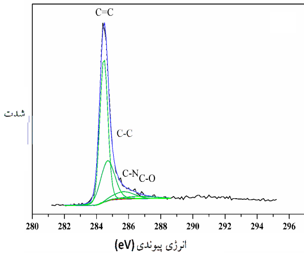
شکل ۷. طیف XPS با قدرت تفکیک بالا بر روی پیک C1s نمونه عملیات حرارتی شده در دمای 850^{\circ}\text{C}
