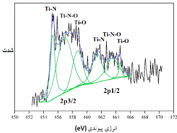
شکل ۸. طیف XPS با قدرت تفکیک بالا بر روی پیک Ti2p نمونه عملیات حرارتی شده در دمای 850^{\circ}\text{C}
