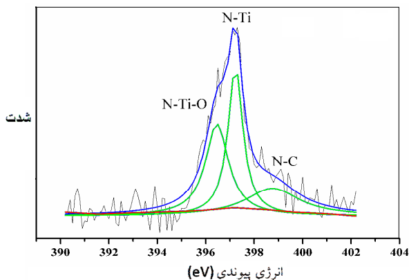
شکل ۹. طیف XPS با قدرت تفکیک بالا بر روی پیک N1s نمونه عملیات حرارتی شده در دمای 850^{\circ}\text{C}
