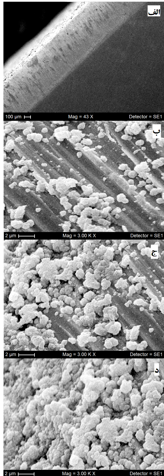
شکل ۷. تصاویر میکروسکوپ الکترونی رویشی مربوط به فصل مشترک پوشش/ زیرلایه و مقادیر مختلف میکروکپسول. (الف) فصل مشترک پوشش/ زیرلایه، (ب) ۰/۰۱ درصد وزنی میکروکپسول، (ج) ۰/۰۰۵ درصد وزنی میکروکپسول، (د) ۰/۰۱ درصد وزنی میکروکپسول.
