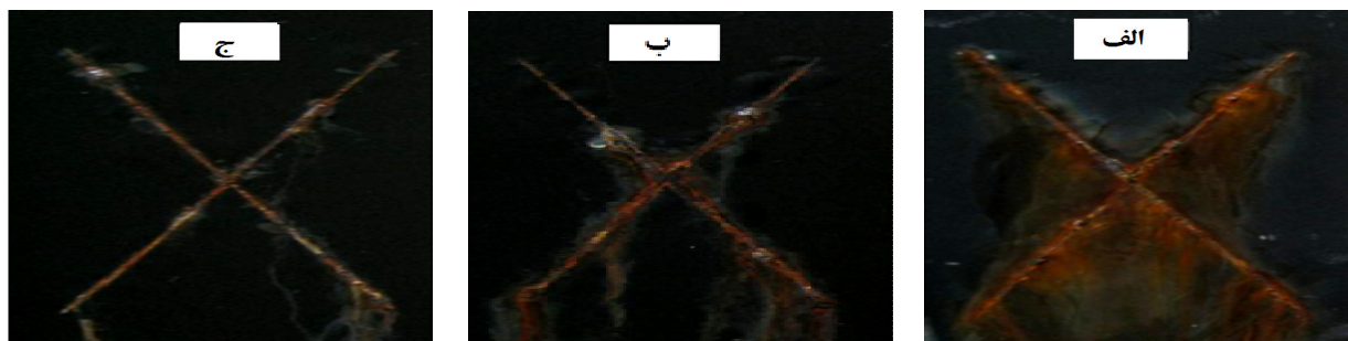
شکل ۹. تصویر پوشش‌های خراش‌دار بعد از ۳۰ روز غوطه‌وری در محلول ۵ درصد کلرید سدیم. الف) نمونه‌ی کنترل، ب) نمونه‌ی شامل ۰/۰۵ درصد وزنی میکروکپسول، ج) نمونه‌ی شامل ۰/۰۱ درصد وزنی میکروکپسول.
