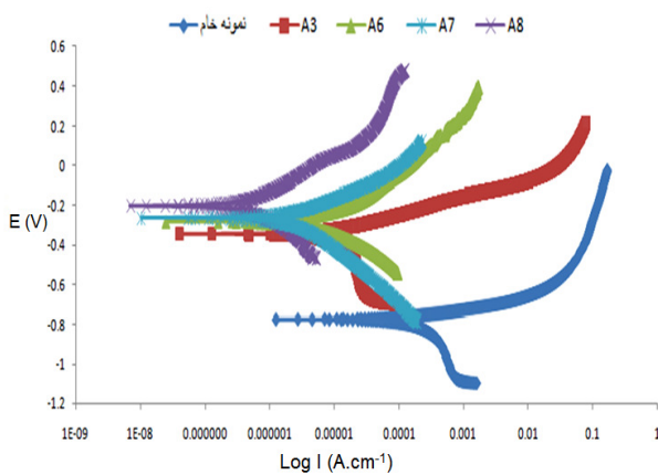
شکل ۸. منحنی‌های پلاریزاسیون تافل برای نمونه‌های بدون پوشش و پوشش‌دهی شده همراه با مقادیر مختلف میکروکپسول.
