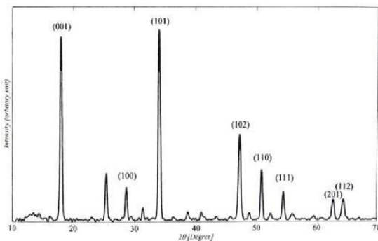
شکل ۴. طیف XRD از نانوپودر هیدروکسید کلسیم، تهیه شده به روش هیدروترمال [۵]
