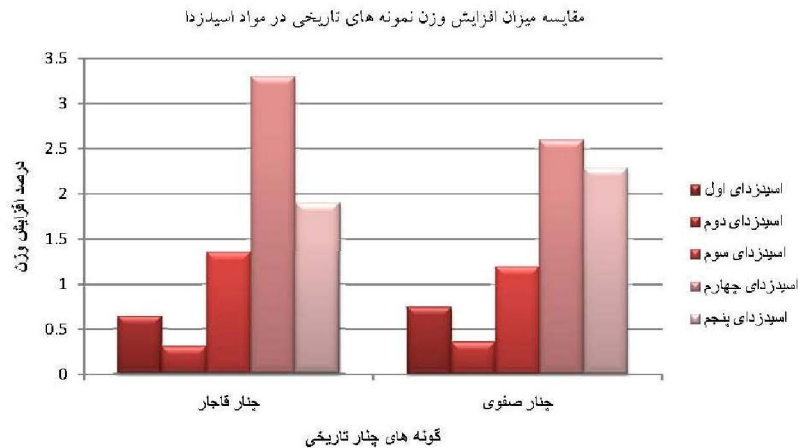
شکل ۱۰. نمودار مقایسه درصد میزان افزایش وزن نمونه‌های تاریخی، در مواد اسیدزدا
